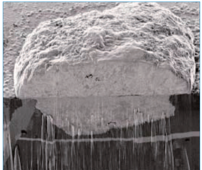
図2 (Fe, Cr) 2 O 3 の外側のCrの消費によって、内側と外側の両方に酸化物が生成され、Fe 2 O 3 が迅速に形成されます。(Competence Centre for High Temperature Corrosion, Professor Lars-Gunnar Johansson, Chalmers Univ. of Technol. 提供)
